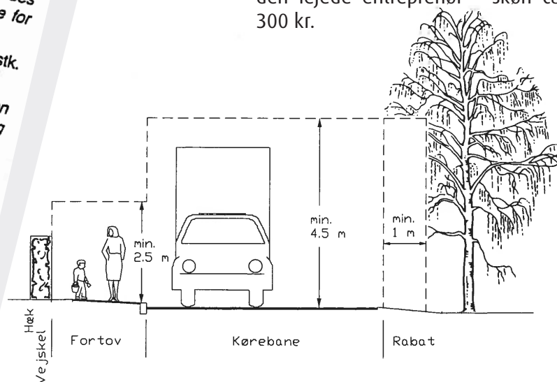
Tværsnit af vej
