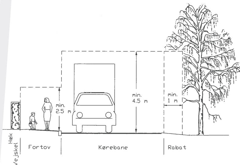
Tværsnit af vej
